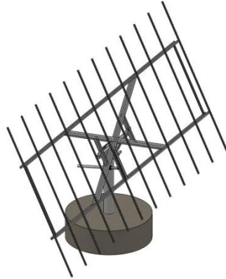
DEGERtraker 7000NT
